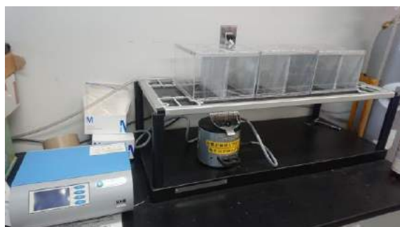
図 1. Dynamic Plantar Aesthesiometer 37540。ラットの足底を器械刺激し、逃避閾値を測定する。
